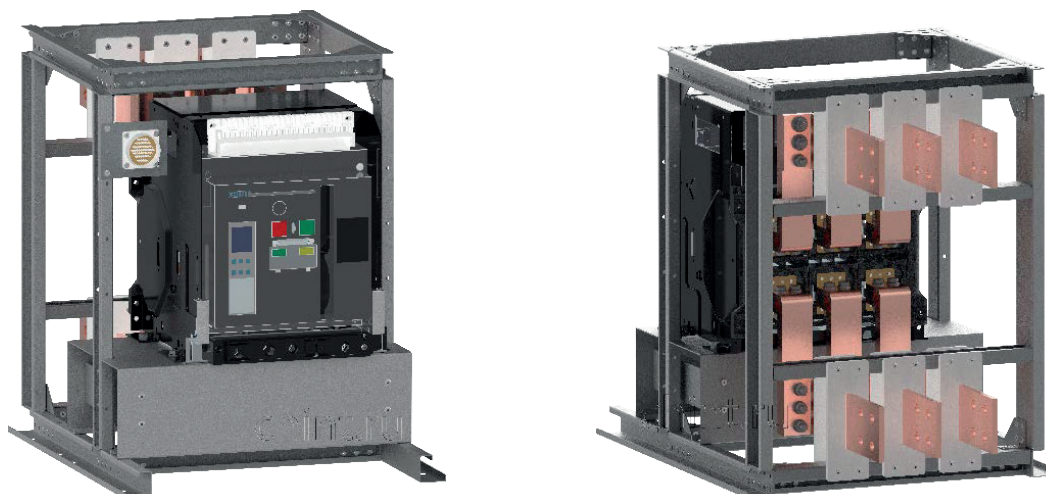
Рис. 1. Основные элементы БЗАВ
